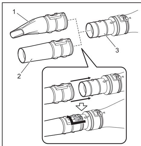
► 1. Boquilla plana 2. Boquilla de extensión 3. Tubo adaptador
